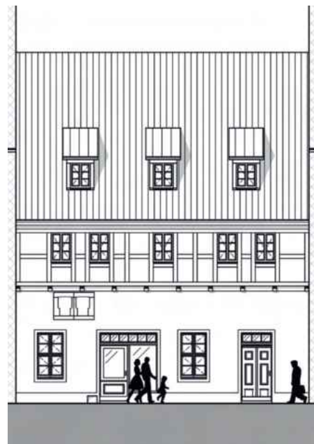
Entwurf Hohe Straße 19 Straßenansicht
