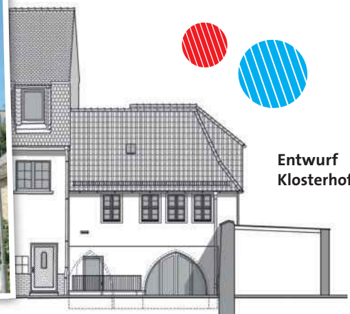
ANSICHT OSTEN
